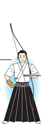
胴造り
